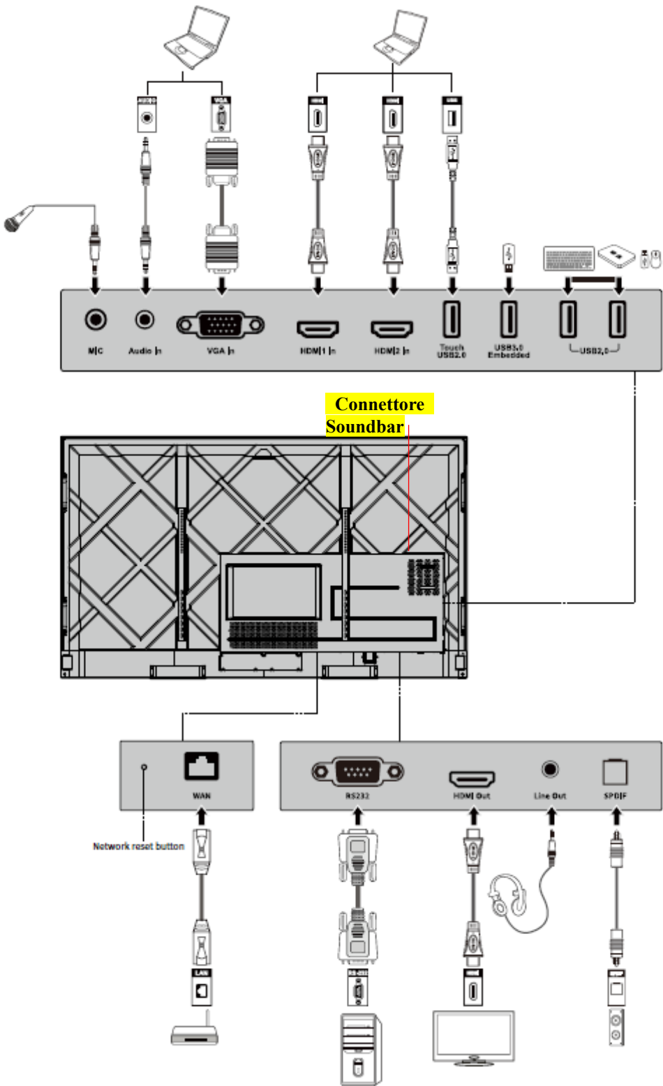
(绘图要求: 增加 TS Series Soundbar 接口连接示意图, 参照 19 款商务中端)
